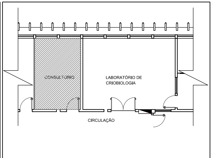
03 ÁREA DE AMPLIAÇÃO - LABORATÓRIO DE CRIBIOLOGIA S/ ESC.
