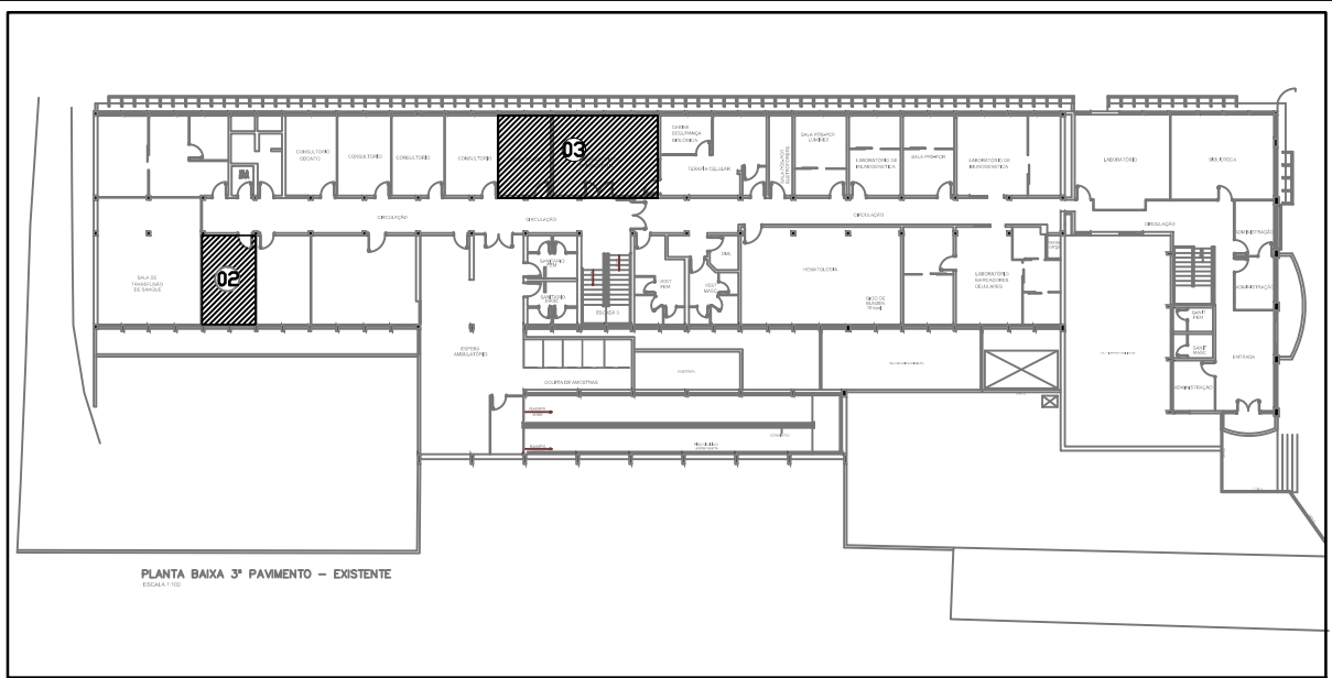
LOCALIZAÇÃO - LABORATÓRIO DE CRIBIOLOGIA, SEGUNDO PAVIMENTO, HEMOSC COORDENADOR S/ ESC.
