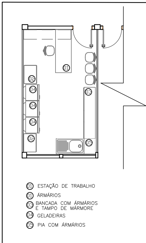
02 NOVO LAYOUT DE MOBILIÁRIO - FARMÁCIA S/ ESC.
